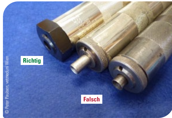
Abb. 7: Bolzenschussgeräte Bauart „Blitz“
